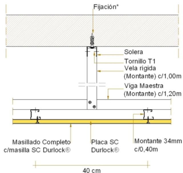
Detalle corte transversal por montantes cada 40cm.
